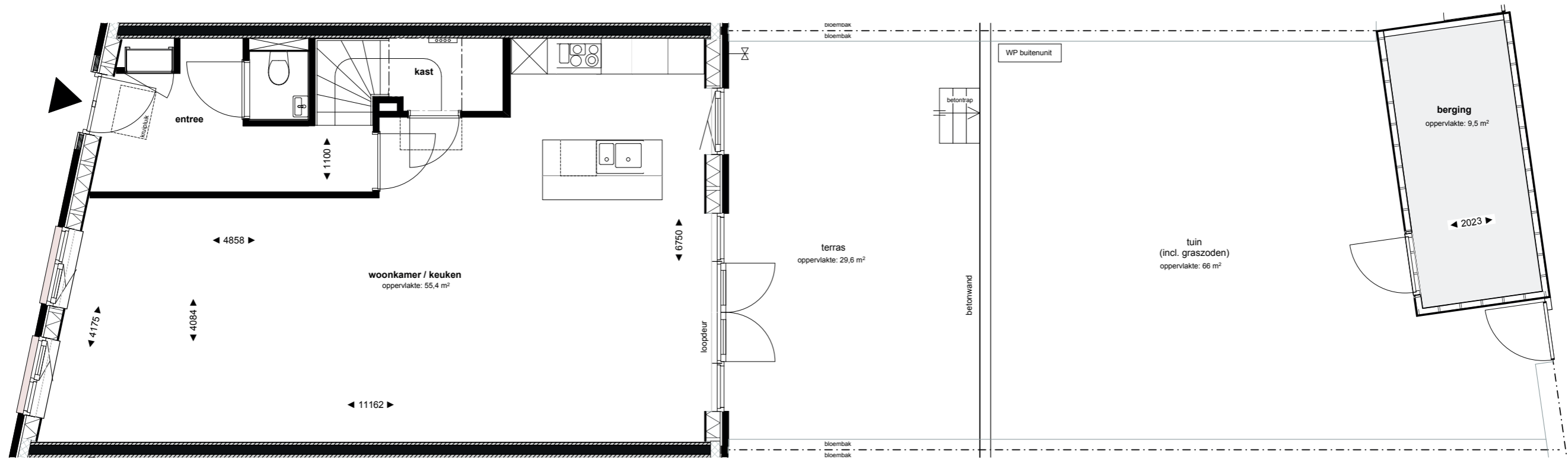
Begane grond
