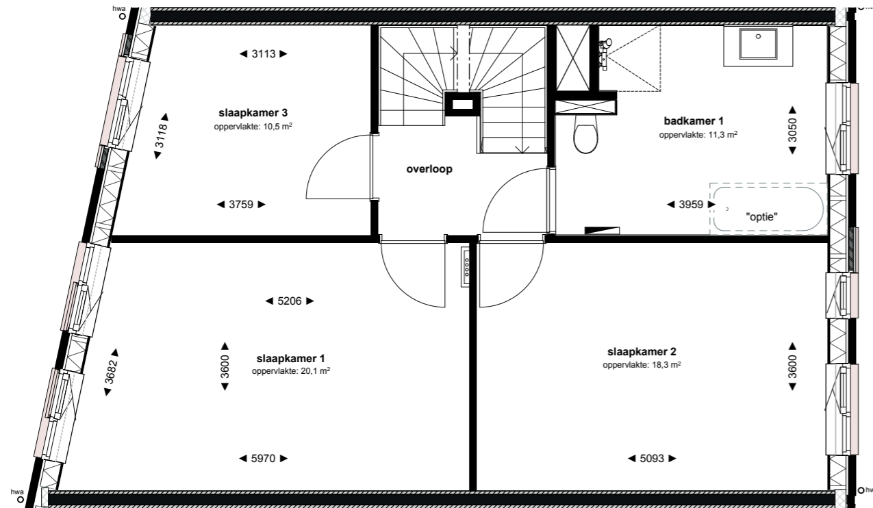
Eerste verdieping
