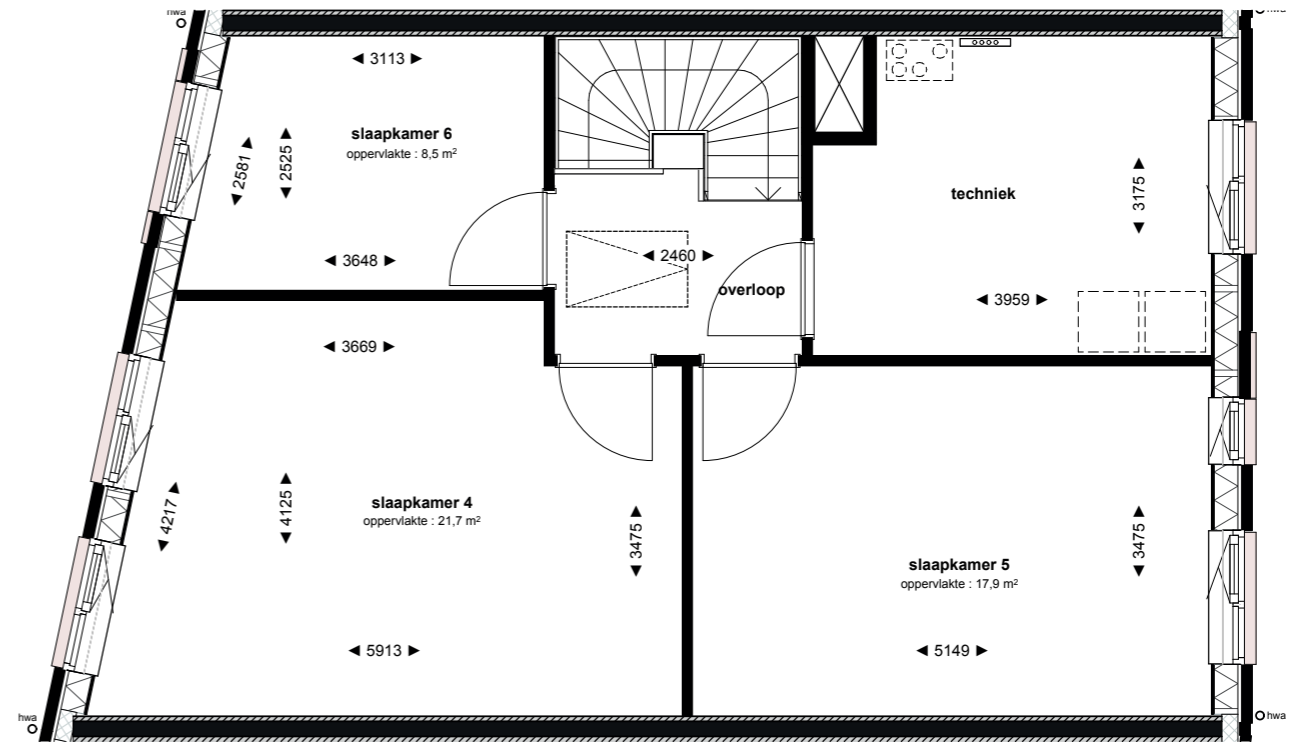
Tweede verdieping
